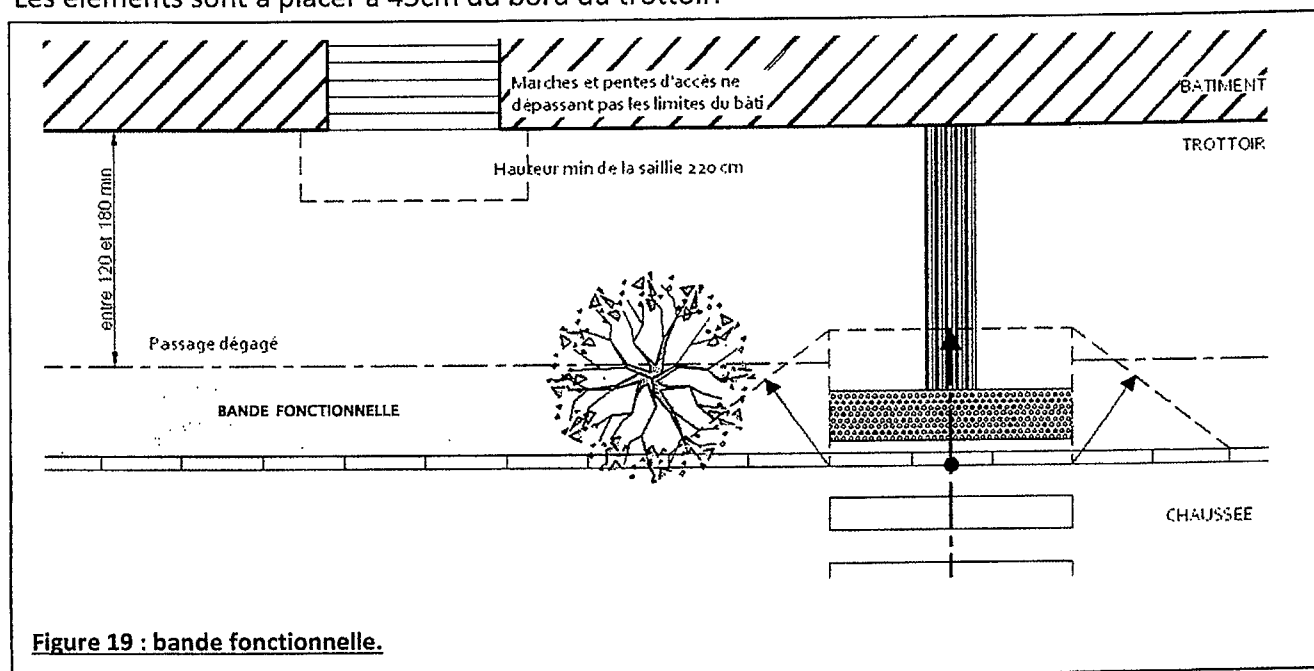
Figure 19 : bande fonctionnelle.
